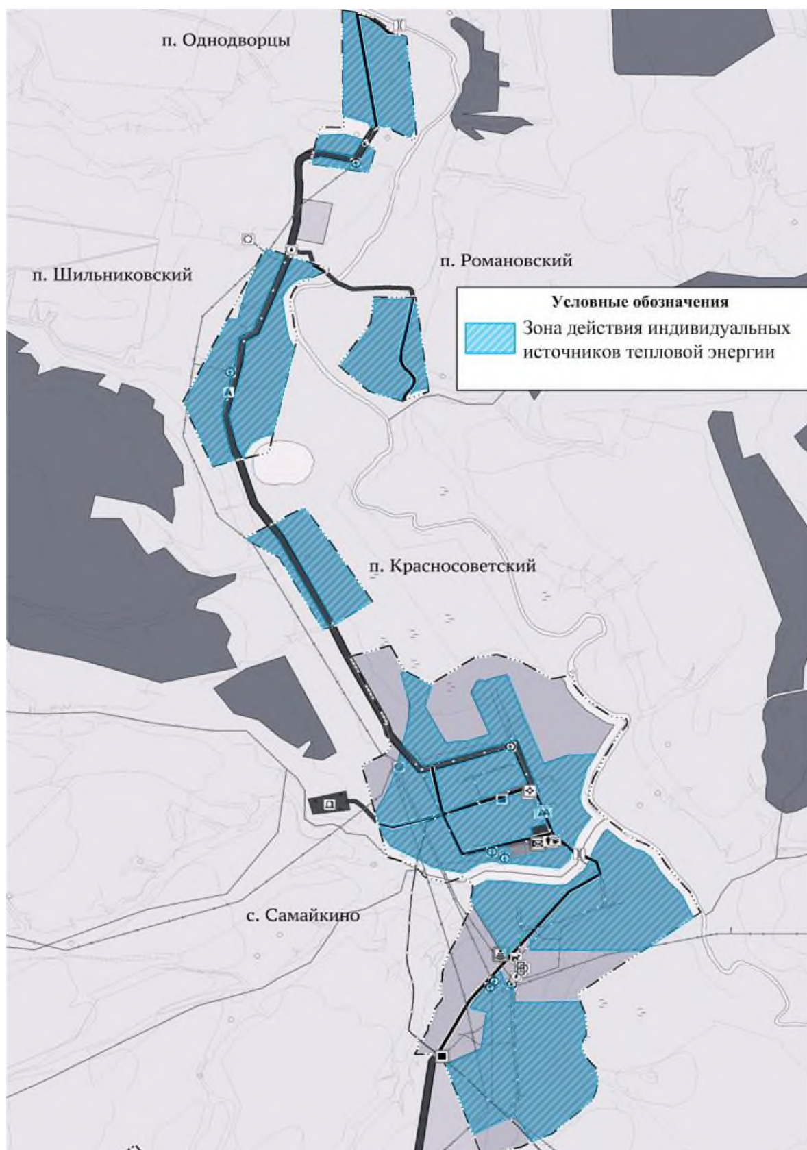
Рис. № 8 - Существующие и перспективные зоны действия индивидуального теплоснабжения территориях с. Самайкино, п. Красносоветский, п. Шильниковский, п. Романовский, п. Одинодворцы (развитие жилой зоны планируется в существующей застройке)
